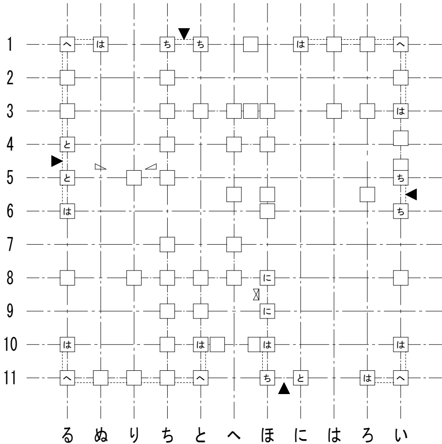
1 階柱壁伏図
